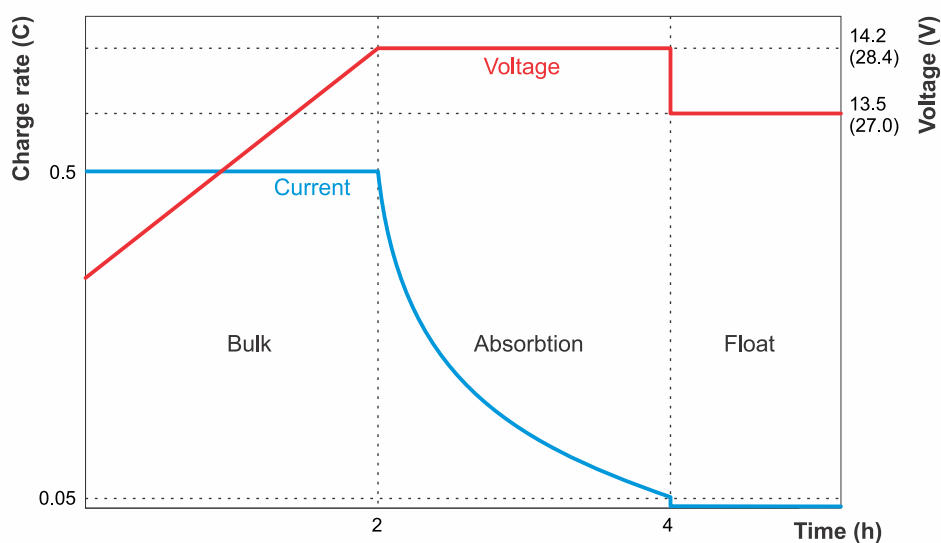
Laddningstabell litiumbatteri
